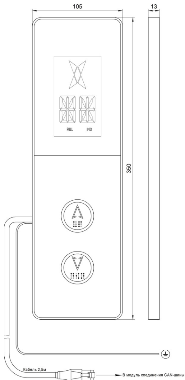
Рис.1 Внешний вид Вызывной пост МАЛАХИТ (жгут RJ45) НШЕК.468381.100
